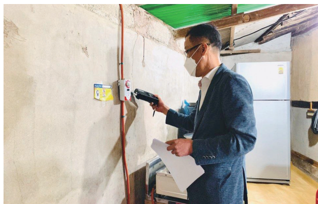
2-2. 안전시설 점검(무안군 일대) [한국가스안전공사 전남서부지사]
